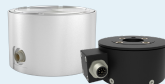
6軸 カトルク 力: 11.2~22.5K lbf トルク: 8.85 lbf-in~88.5K lbf-in 力: 50 N~100K N トルク: 1 Nm~10K Nm
