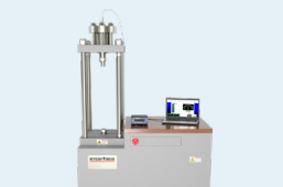
GS-SYS Gold Standard® 校正システム ロードフレーム 最大容量100K lbf
