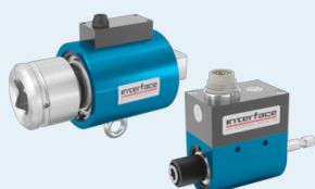
T12/T15 スクエアドライブ 0.88 lbf-in ~ 177K lbf-in 0.1 Nm ~ 5K Nm
